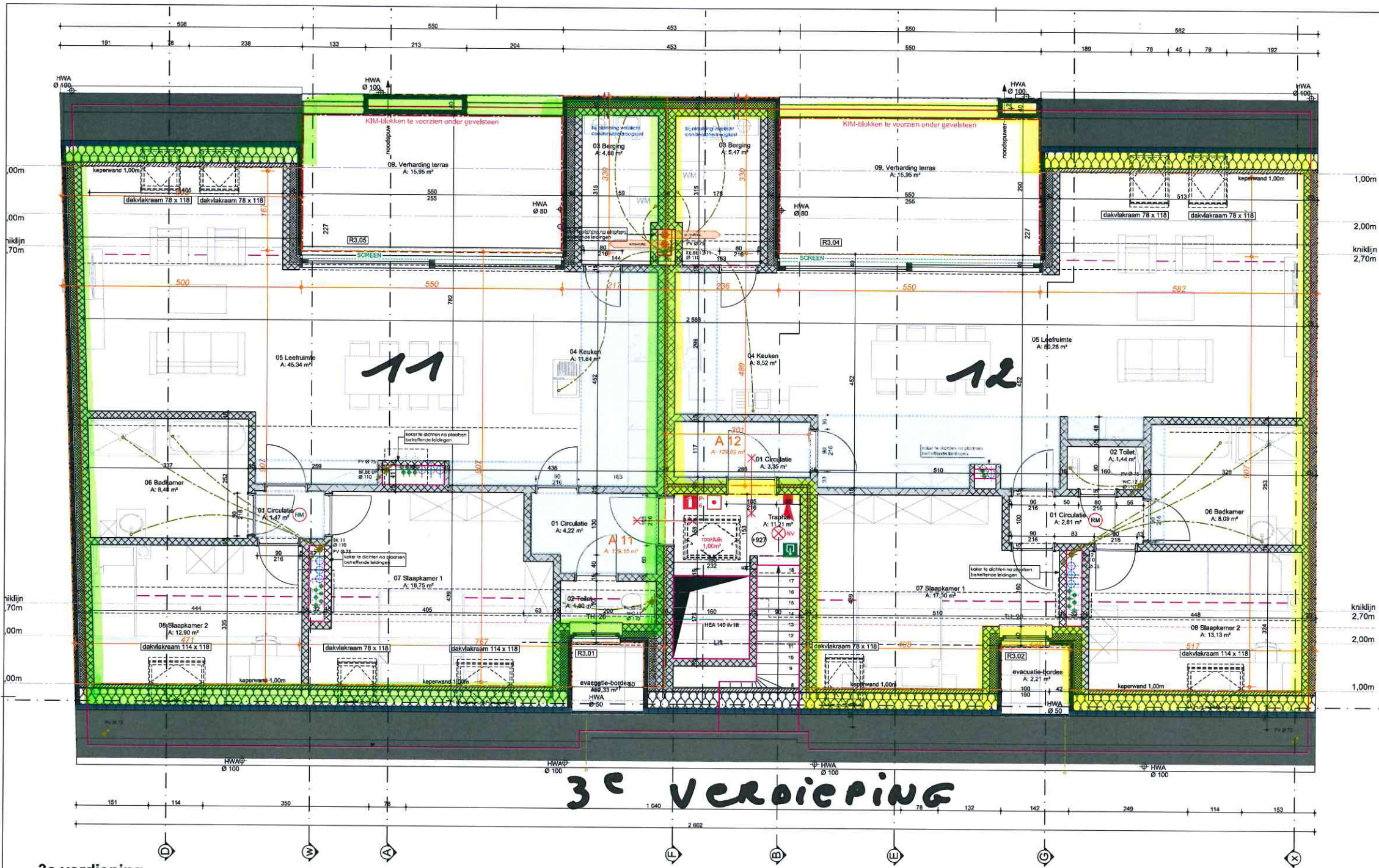
3e verdieping 1:50
