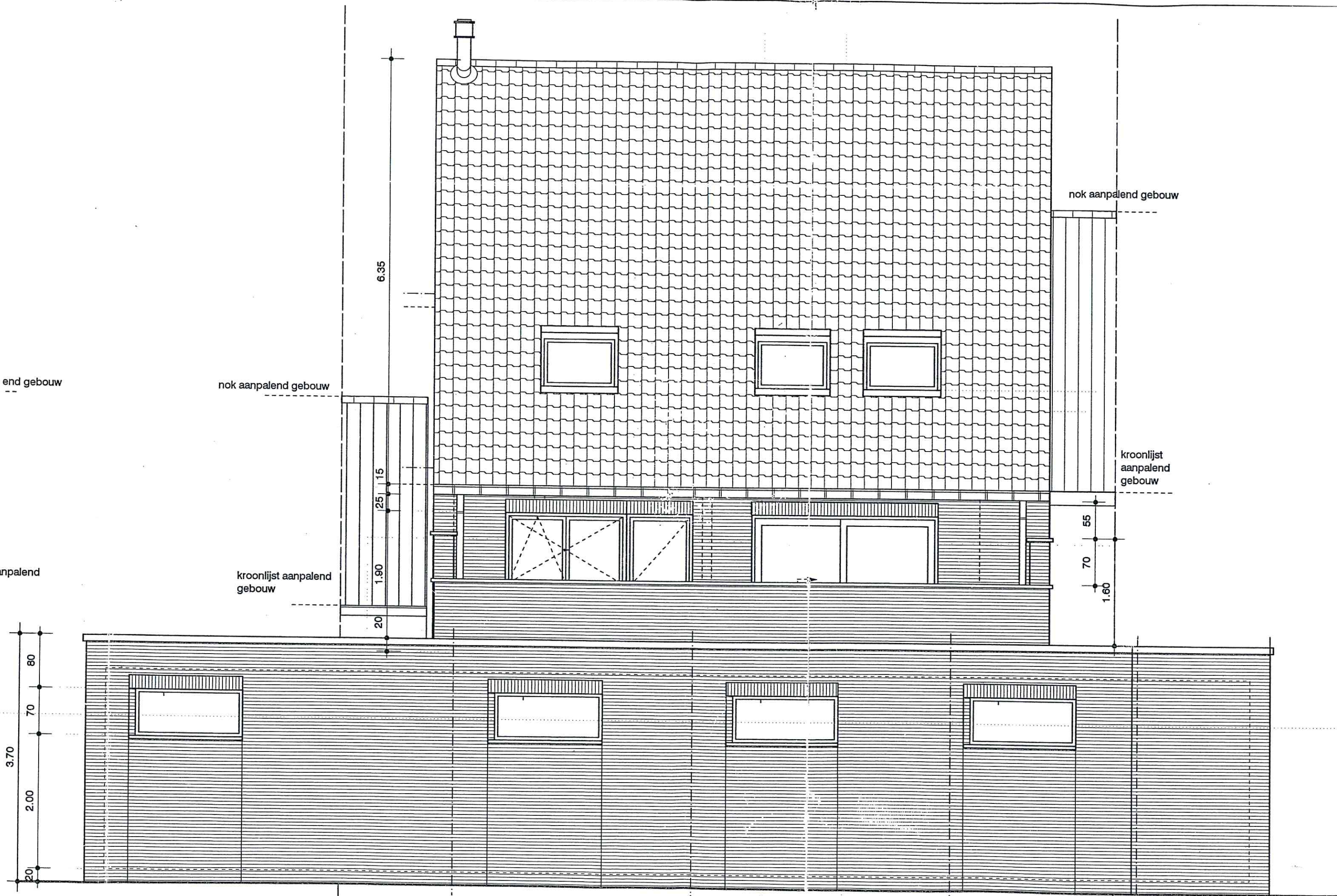
ACHTERGEVEL 1/50
